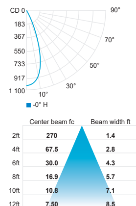
HO flood 39° (3000K, 90CRI)
