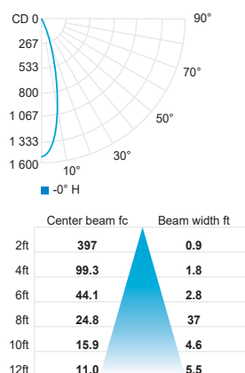
HO medium 26° (3000K, 90CRI)
