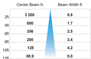
3000K - HO - 80 CRI - 45.5W - Spot 20°
