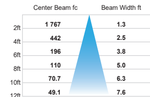
3000K - HO - 80 CRI - 45.5W - Flood 35°
