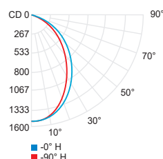
MO Microprismatique (3000 K, 90 CRI)
