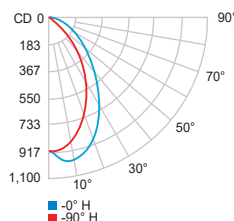
3000K - HO - 80 CRI - 29W - Wall Washer
