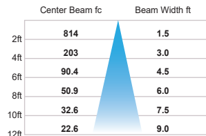
3000K - HO - 80 CRI - 29W - Flood 40°
