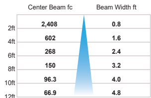
3000K - HO - 80 CRI - 29W - Spot 20°
